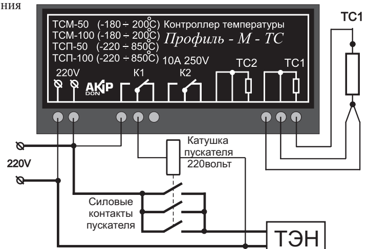
Рис. 3. Монтажная схема системы. Применяется при условии, что мощность нагревательного элемента превышает 1,5 киловатта. Тип пускателя определяется мощностью нагрузки (ТЭНов).
