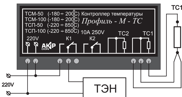
Рис. 2. Монтажная схема системы. Применяется при условии, что мощность нагревательного элемента не превышает 1,5 киловатта.
