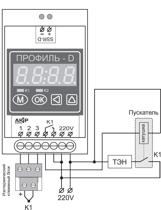
Рис. 3. Схема системы с использованием промежуточных реле или пускателей.
