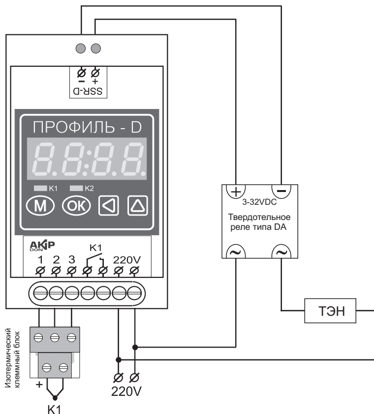
Рис. 4. Схема системы с использованием твердотельных реле. При использовании твердотельных реле необходимы радиаторы для их охлаждения.
