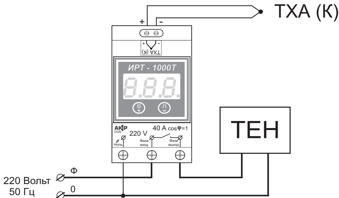
Рис. 1. Схема монтажа прибора.
