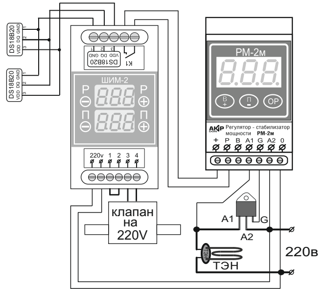
Рис. 3. Вариант подключения прибора в режиме P3. Терморегулятор t2 прибора ШИМ-2 используется для управления режимом разгона PM-2м.
