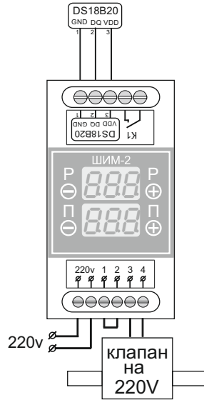
Рис. 2. Вариант подключения прибора в режиме P2. Старто-стопы для отбора формирует встроенный термоконтроллер t1.
