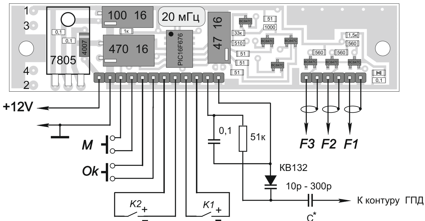
Рис..2 Схема подключения шкалы к трансиверу.
