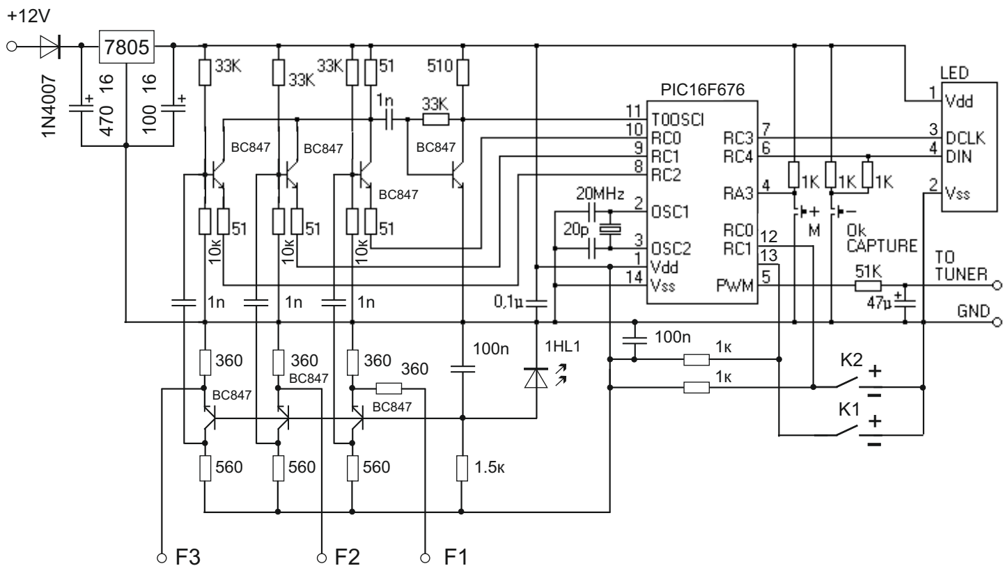
Рис..1 Принципиальная схема шкалы
